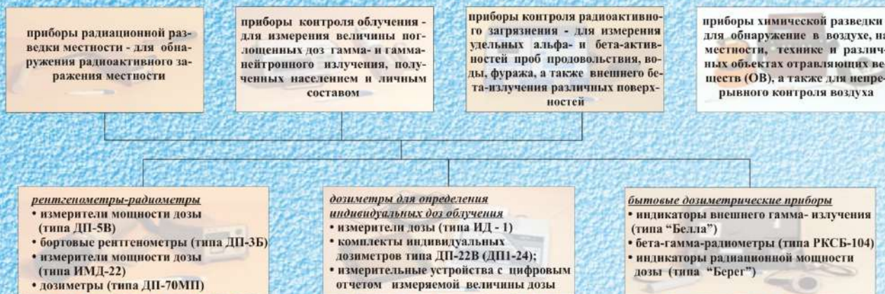
Краткая характеристика переносных радиометрических и дозиметрических приборов
