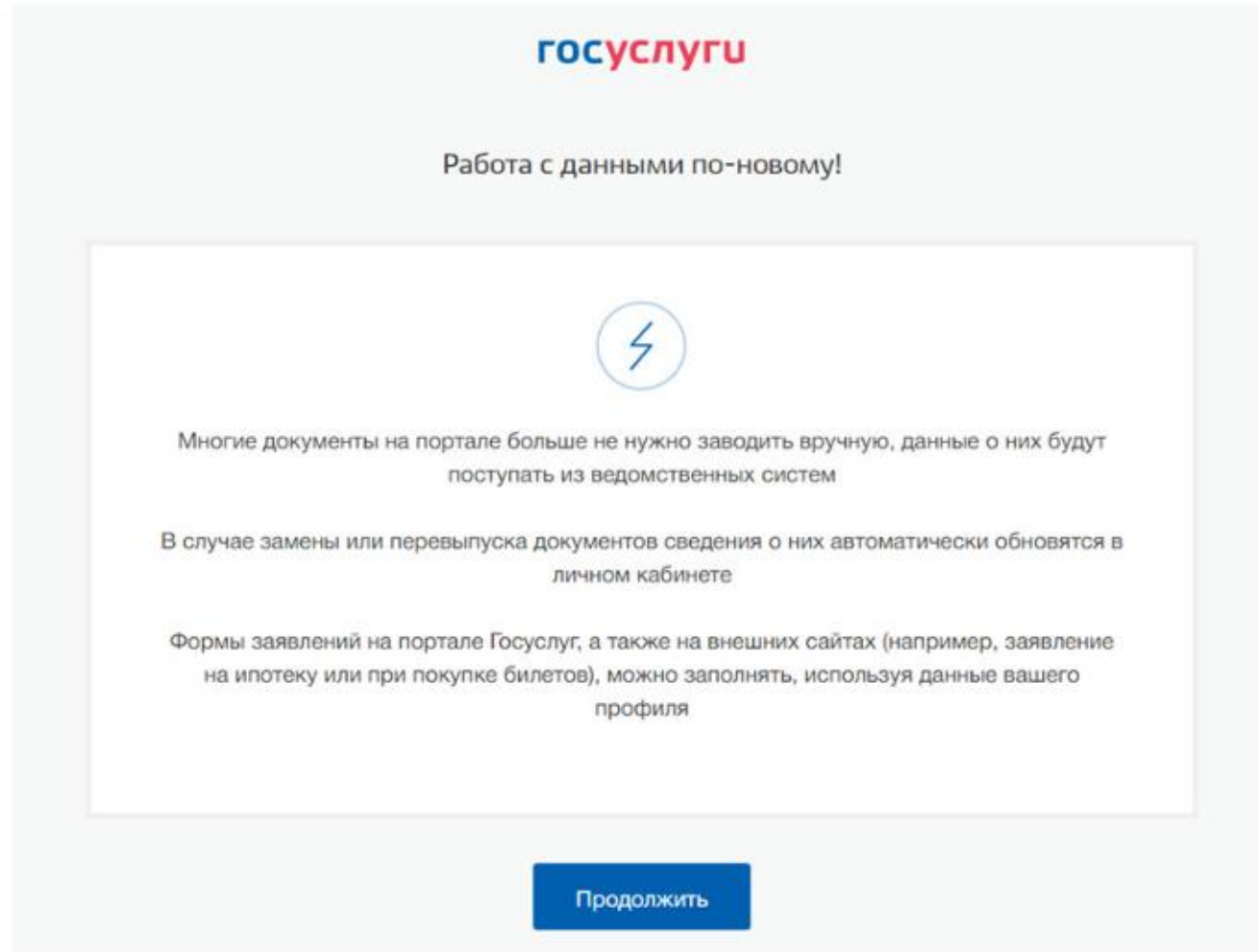
Рисунок 7 – окно информирования
